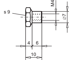
STEP NUT M4
