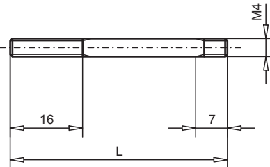
STUD M4xL
