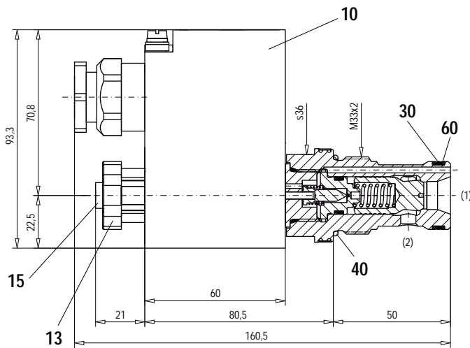
2/2-way version, «normally open» [CD]
